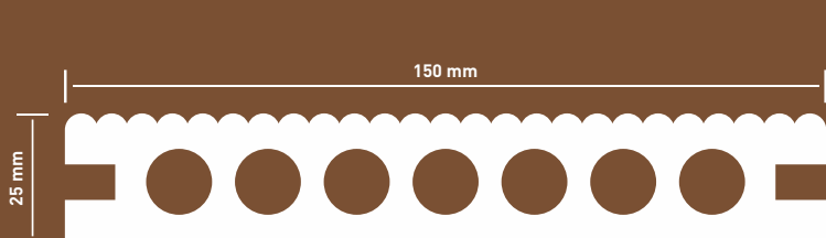
terasové prkno, délka 200 a 400 cm
